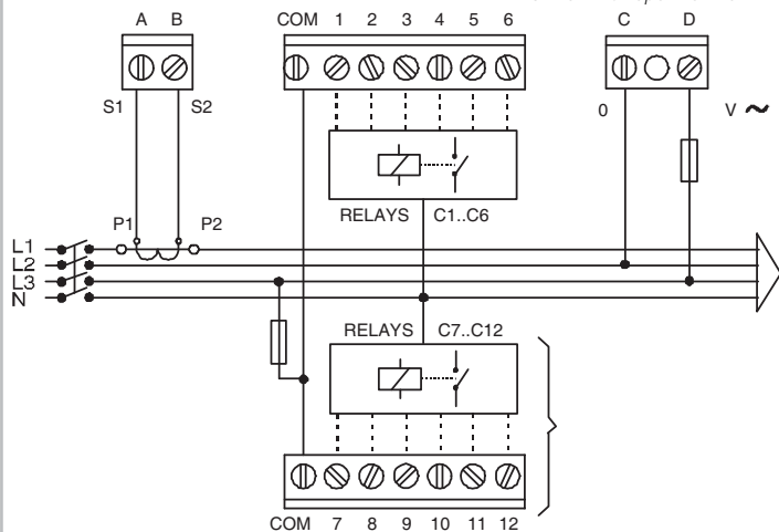
Рис. 4.2 Схема подключения MCE12ADV
