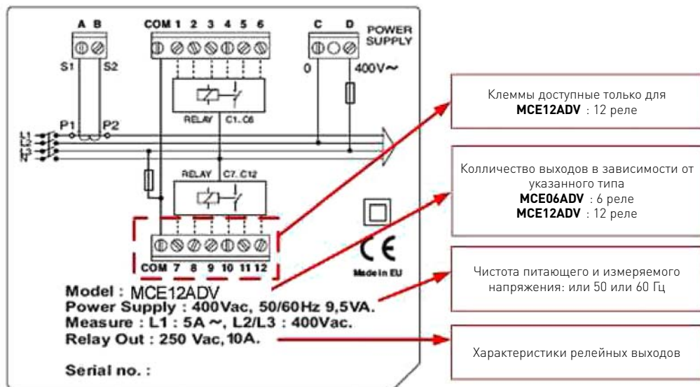
Рис. 1.1.- этикетка задней панели
