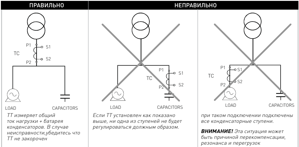
Рис. 4.1.- Размещение трансформатора тока (ТТ)
